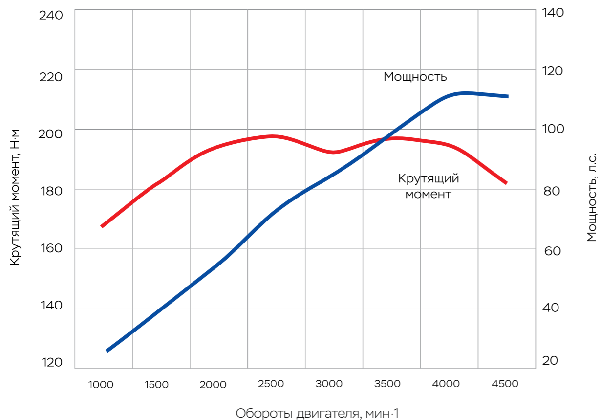
ЗМЗ-40911 - современный 16-клапанный двигатель ЕВРО-2 объемом 2,7 л и мощностью 112,2 л.с.
